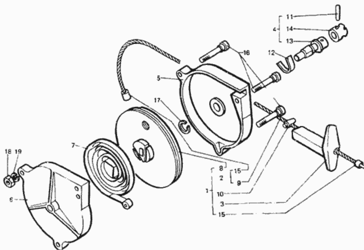
Рис. 57. Стартер ручной ПД8-1022010
